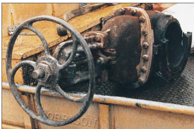
Rysunek 6. Żeliwne zasuwy rozerwane na skutek uderzeń wodnych w rurociągach parowych.
