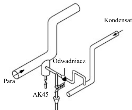
Rysunek 5. Sposób wykorzystania zaworu odwadniająco-rozruchowego AK45
