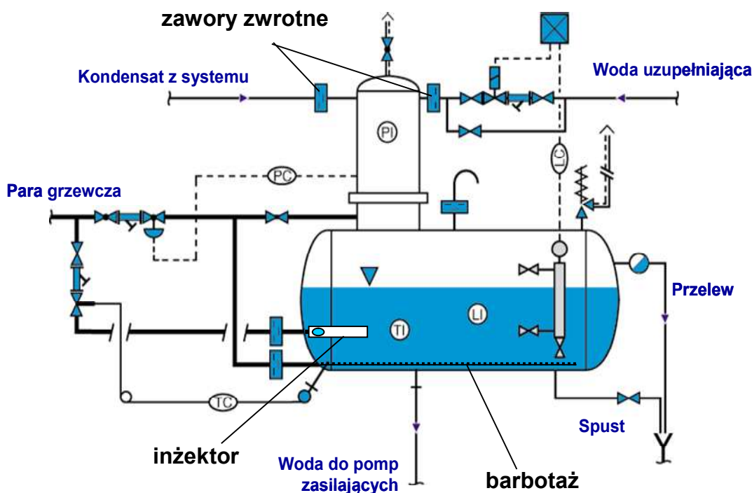
Rysunek 15. Zbiornik wody zasilającej z pełnym odgazowaniem termicznym + osprzęt.
