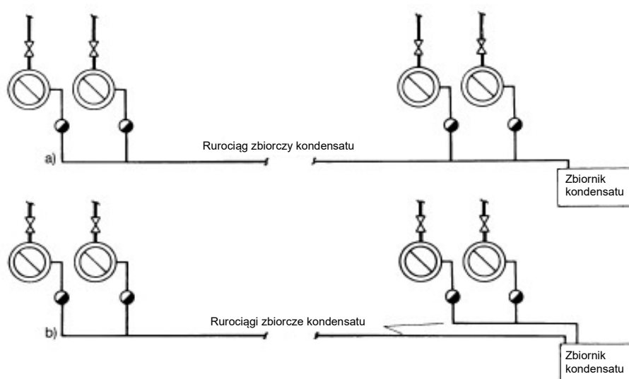
Rysunek 11. Mieszanie kondensatu z odległych odbiorników.
